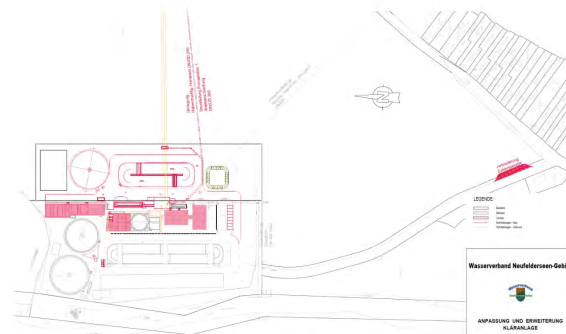
Bild: Auszug Lageplan Baumaßnahmen Kläranlage (BA18)
